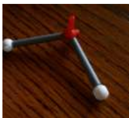
H 2 O
